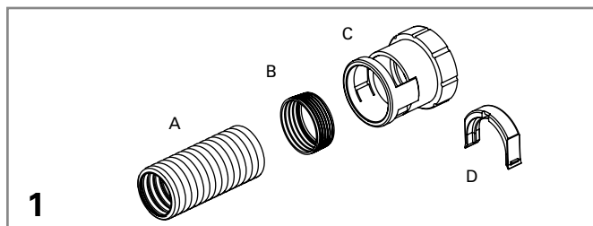
A. Gaine B. Joint d'étanchéité Ex (jaune) C. Raccord D. Clip ovale
