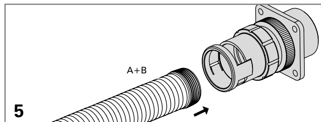
Rohr mit Dichtkappe (A+B) so weit in den Fitting einstossen, dass die Dichtkappe nicht mehr im Sperrenfenster sichtbar ist.
