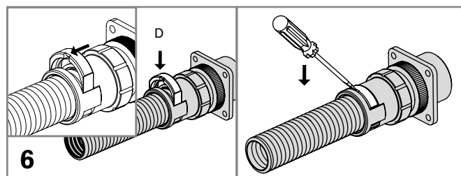
Inserte el clip oval (D) en la hendidura de fijación hasta su encaje. La muesca para el destornillador debe apuntar hacia el tubo. Para abrirlo utilice un destornillador.
