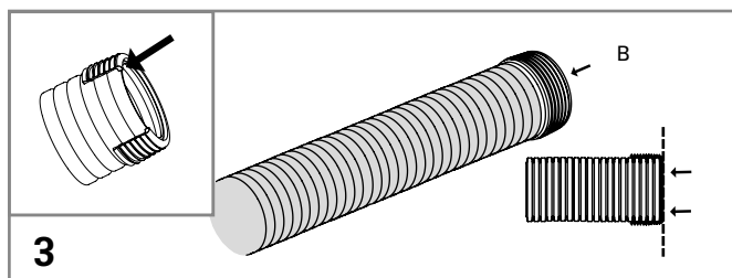
Pousser le joint d'étanchéité (B) complètement sur la gaine pour obtenir l'étanchéité IP68.
