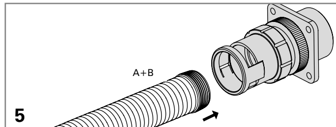
Spingere la guaina dotata di guarnizione di tenuta (A+B) nel connettore finché la guarnizione non sarà più visibile nell'apposita apertura.
