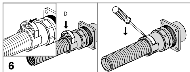
Oval-Sperre (D) in das Sperrenfenster einsetzen und einrasten. Die Schraubenzieher-Öffnungsnut muss rohrrseitig positioniert sein. Wieder öffnen mittels Schraubenzieher.
