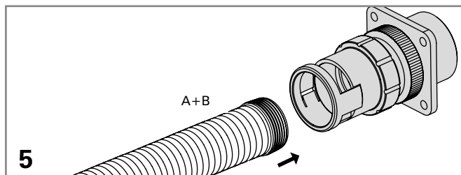
Pousser la gaine avec le joint d'étanchéité (A+B) dans le raccord jusqu'à ce que le joint ne soit plus visible dans la fenêtre du clip ovale.
