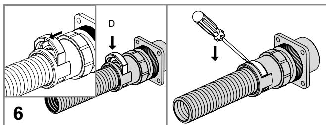
Insérer le Clip ovale (D) dans la fenêtre adéquate et encliqueter. Il faut positionner la fente du clips coté gaine. Pour enlever le clip utilisez un tournevis.
