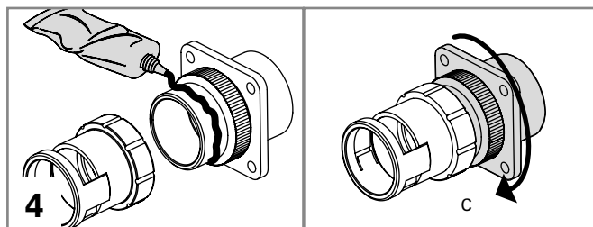
Visser le raccord (C). (Voir les remarques concernant la sécurité).
