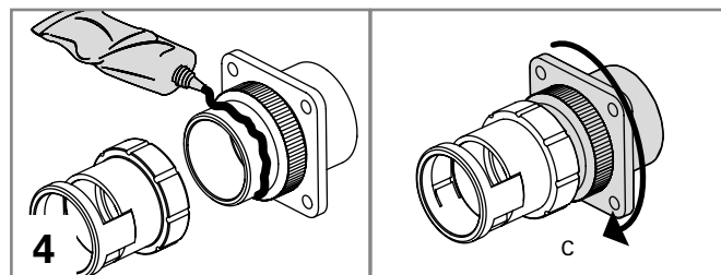
Atornille el racor (C). (Ver observaciones de seguridad).
