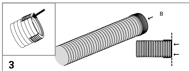
Um die Dichtheit zu gewährleisten, Rohrdichtung (B) ganz auf das Rohr aufstossen.
