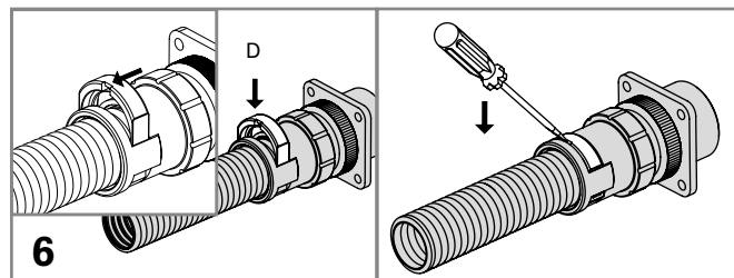
Inserire nell'apertura il dispositivo di bloccaggio ovale (D). Per riaprire utilizzare un cacciavite. Posizionare il cacciavite come raffigurato nell'immagine.
