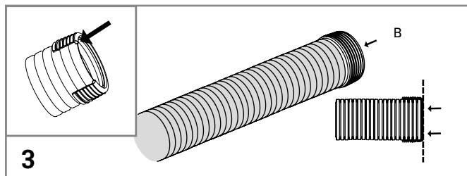
Per la classe di protezione IP68, posizionare la guarnizione di tenuta (B) sulla guaina in modo che risulti completamente inserita.
