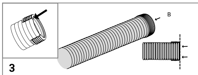
Para obtener una estanqueidad óptima empujar completamente el manguito (B) sobre el tubo.
