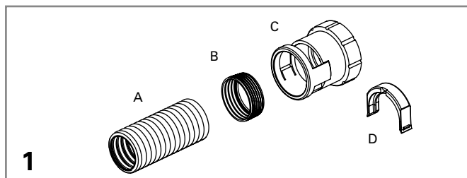
A. Tubo B. Manguito Ex (amarillo) C. Racor D. Clip oval
