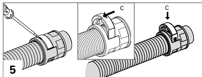
Wieder öffnen mittels Schraubenzieher. Die Schraubenzieher-Öffnungsnut an der Sperre (C) muss rohreseitig positioniert sein.
