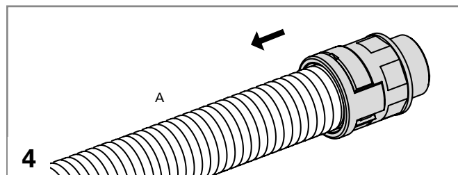
Wellrohr (A) leicht zurückziehen, damit die Verriegelungselemente optimal einrasten.
