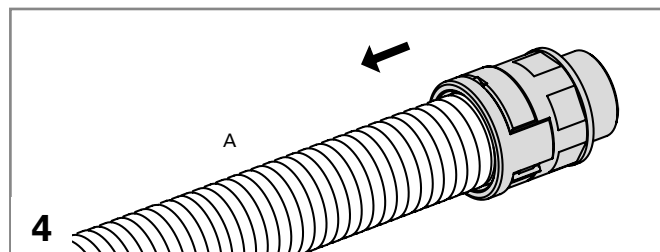
Tirer légèrement sur la gaine (A) pour s'assurer que le mécanisme de verrouillage est bien enclenché.
