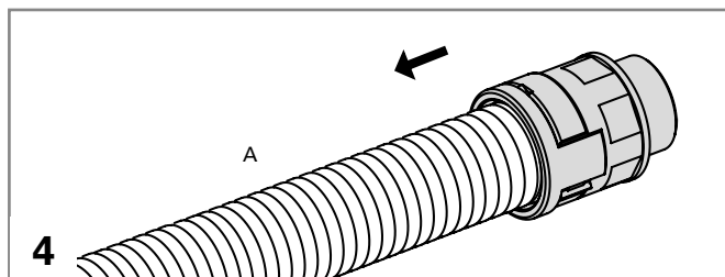
Tirare leggermente indietro la guaina (A) per consentire agli elementi di bloccaggio di innestarsi in posizione.
