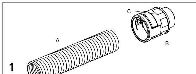
A. Tubo B. Racor C. Clip universal de seguridad
