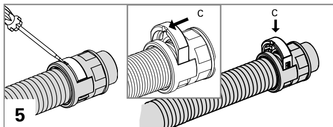
Utilizar un destornillador para abrir. Al volver a montar el clip de seguridad (C), asegurarse de que la ranura para el destornillador queda orientada hacia el tubo.
