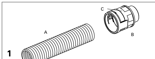
A. Wellrohr B. Anschlussarmatur C. Universal Sicherheits-Sperre
