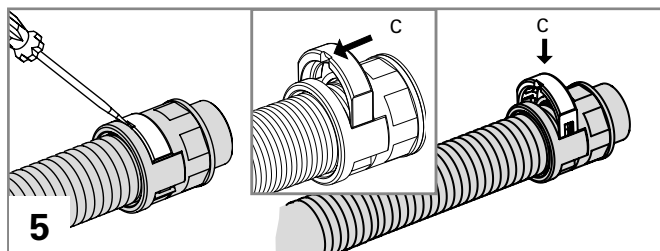
Per riaprire utilizzare un cacciavite. Posizionare il cacciavite come raffigurato nell'immagine.
