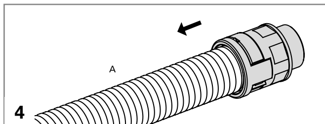
Tirar ligeramente del tubo (A) para asegurarse de que los elementos de bloqueo encajan perfectamente.
