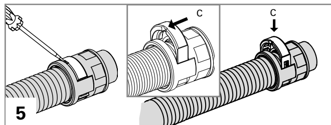
Pour enlever le clip utilisez le tournevis. Il faut positionner la fente du clips (C) côté gaine.
