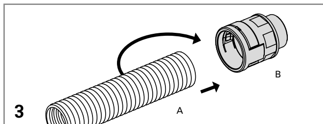
Einstossmontage des Wellrohres (A) mit leichter Drehbewegung. Rohr bis zum Anschlag einstossen.
