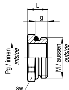
Dimensions Dimensionen
