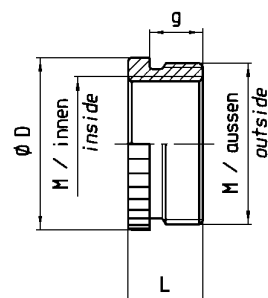
Dimensions Dimensionen
