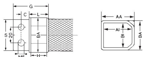
REV NW40 Dimensions Dimensionen
