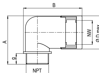
Dimensions Dimensionen
